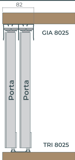
RO 47 VERSATILE Sistema Embutido
