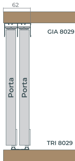
RO 47 - Versatile Sistema Embutido
