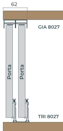
RO 62 UNIVERSAL Sistema Sobreposto
