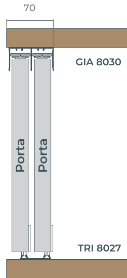
RO 47 VERSATILE Sistema Embutido
