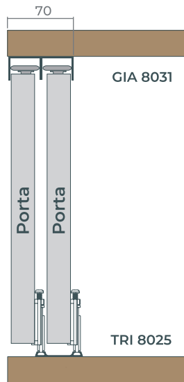
RO 62 UNIVERSAL Sistema Sobreposto
