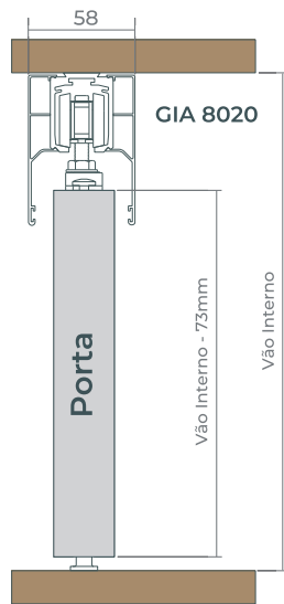
Fixação do trilho no teto
