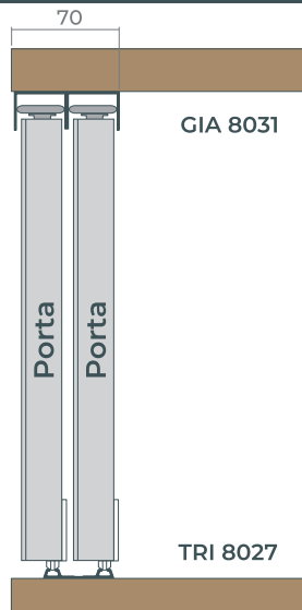
RO 47 UNIVERSAL Sistema Embutido
